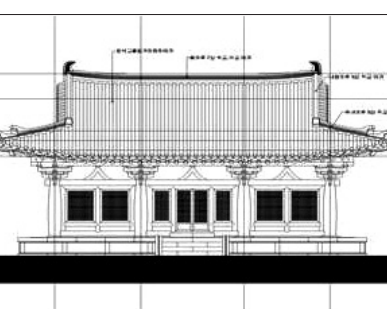
JSA법당 정면도
