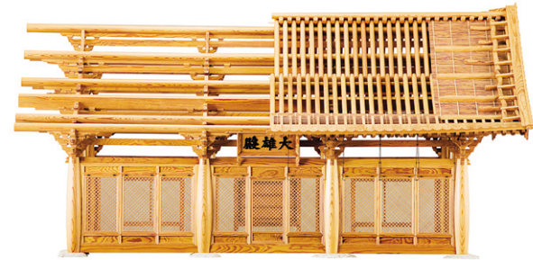
고려시대 대표적 목조건축물인 수덕사 대웅전.
