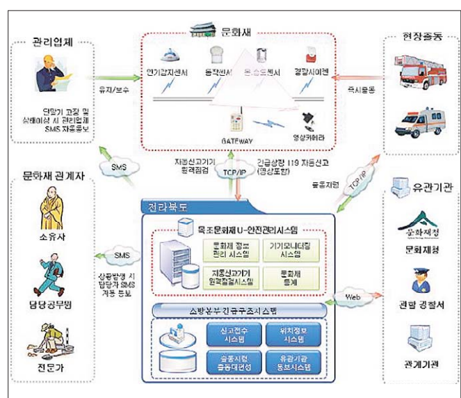
전북도가 구축하고자 하는 u-안전관리시스템 구성도
