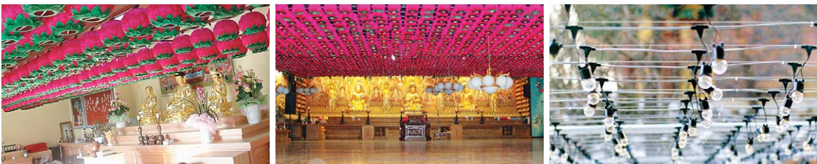
연등 자동 승강장치 _ 대구 장성사
