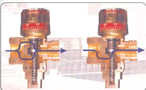
이중유로방식밸브 단일유로방식밸브
