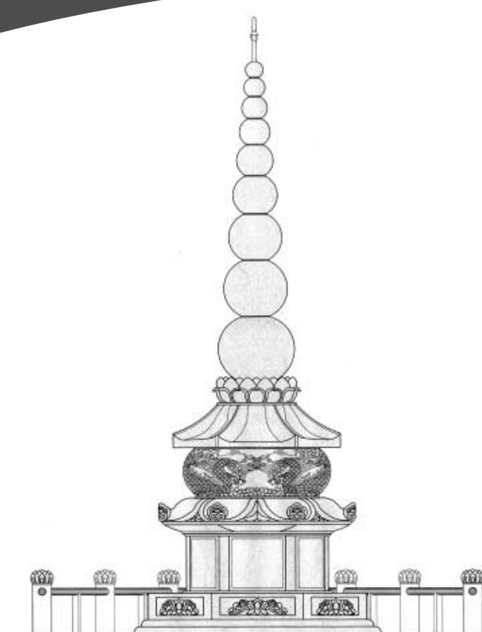
울산지원 도량탑 입면도(9층)
