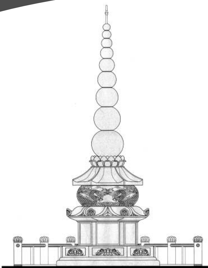
울산지원 도량탑 입면도(9층)
